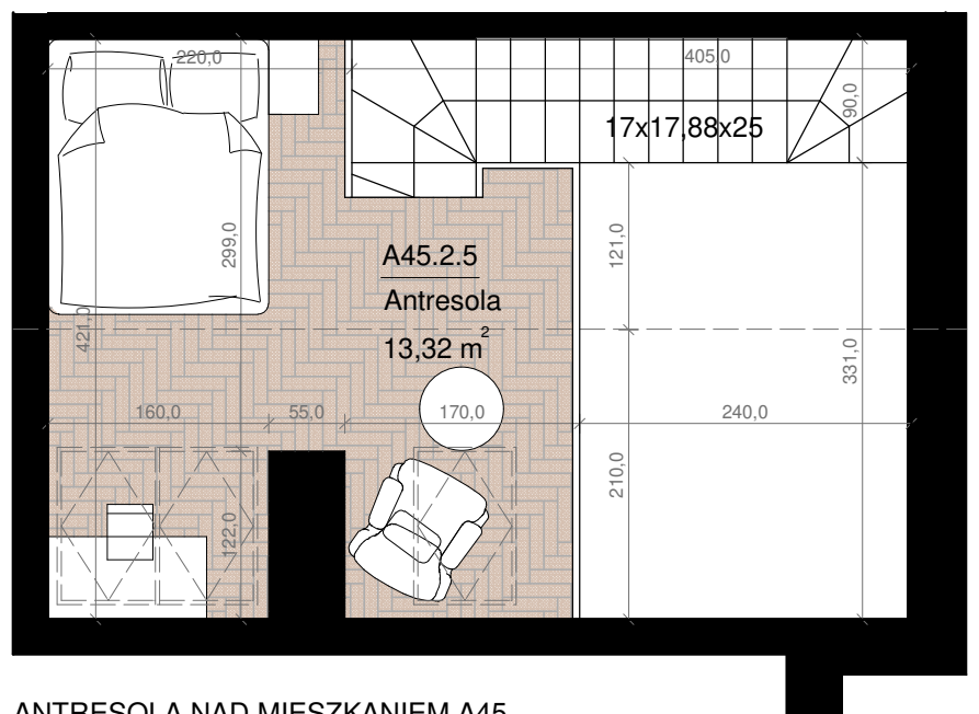
ANTRESOLA NAD MIESZKANIEM A45
